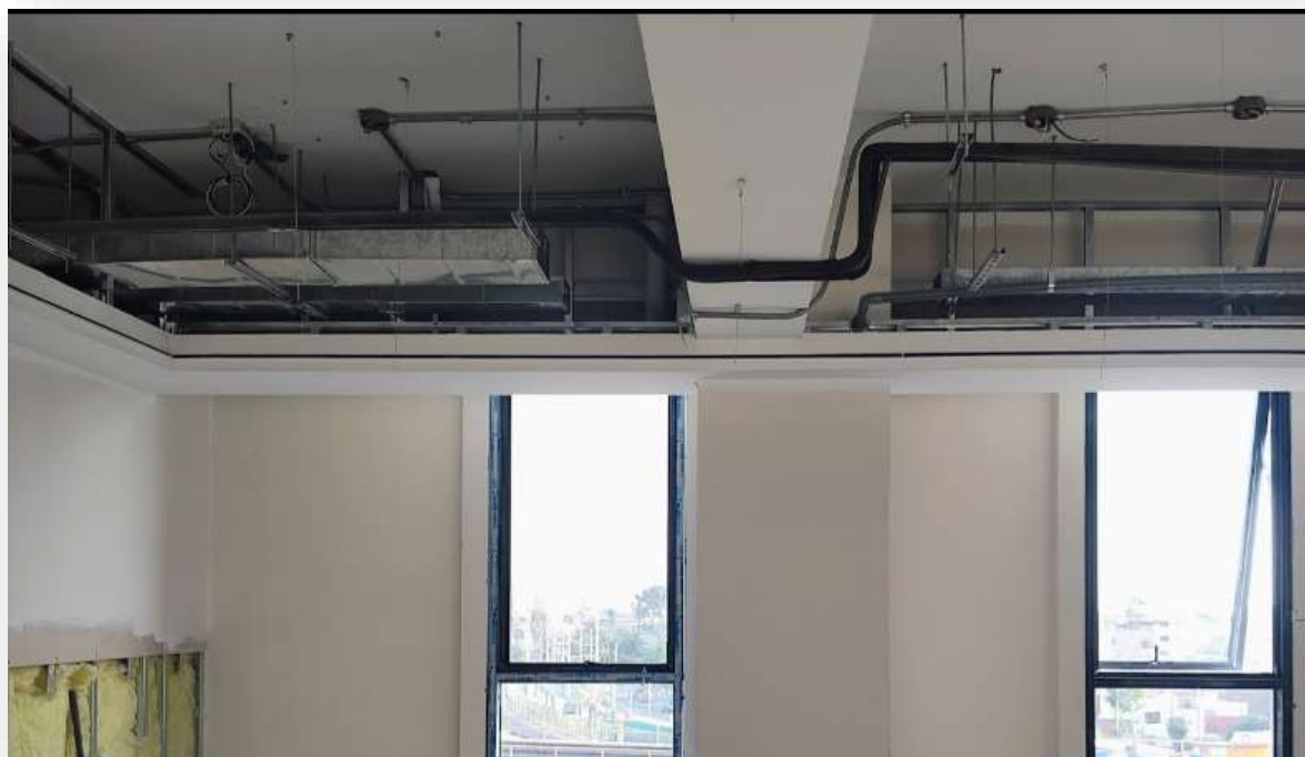
INSTALACIÓN DE TUBERÍA DE COBRE EN TODAS LAS OFICINAS
