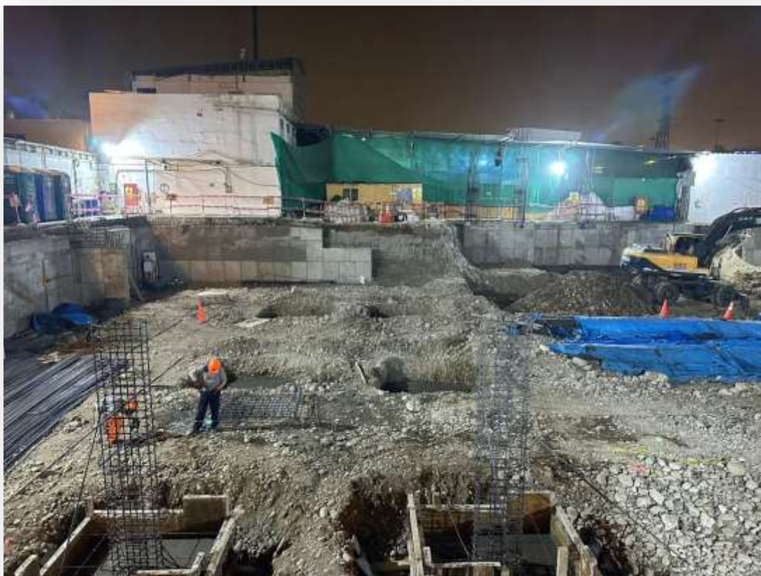
HABILITADO DE ACERO Y ENCOFRADO DE CIMENTACIÓN
