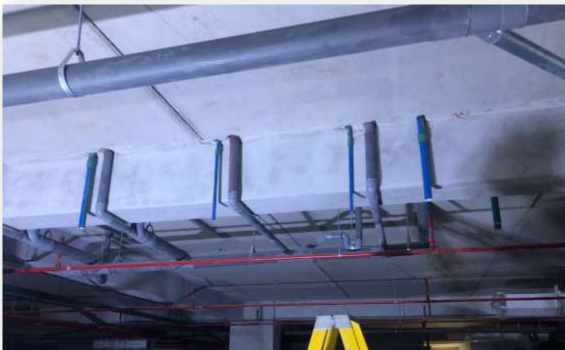
INSTALACIÓN DE TUBERÍAS COLGANTES EN SÓTANO 1
